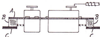
A — servoplade med udskæringer. B — 8-10 mm vibrationsgummi. C — 4 mm krydsfinerstrip, der fastgøres i modellen.
