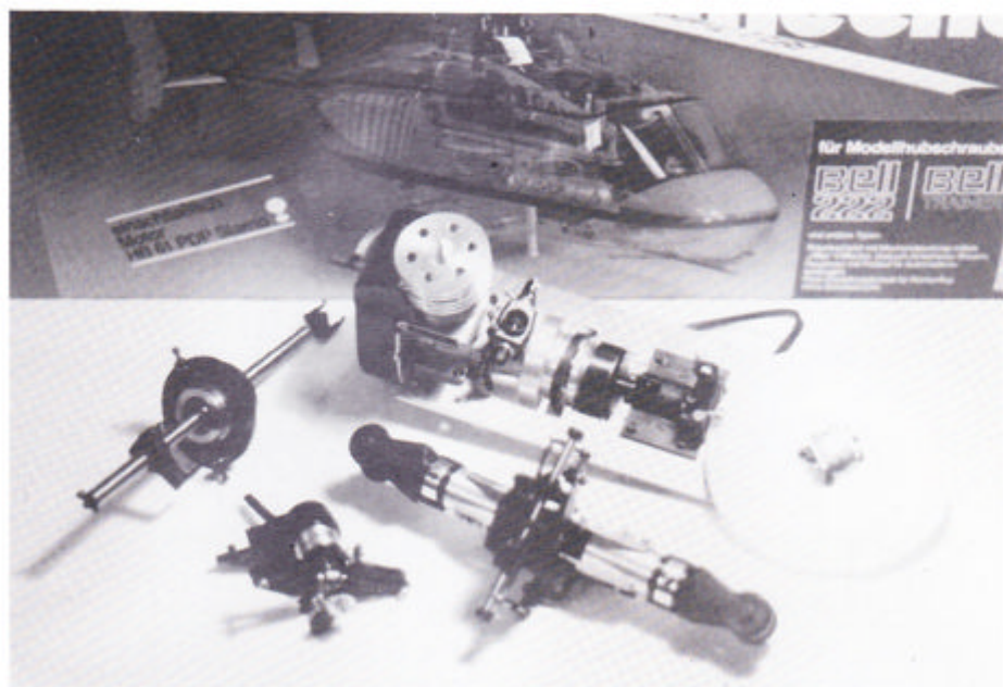
De fire hoveddele fra mekaniksettet. Motoren er monteret med bagmonteret blæser.
