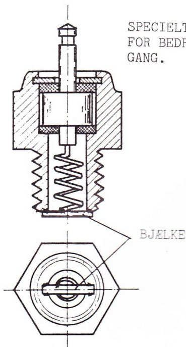
Fig. 3. Bjælkerør.
