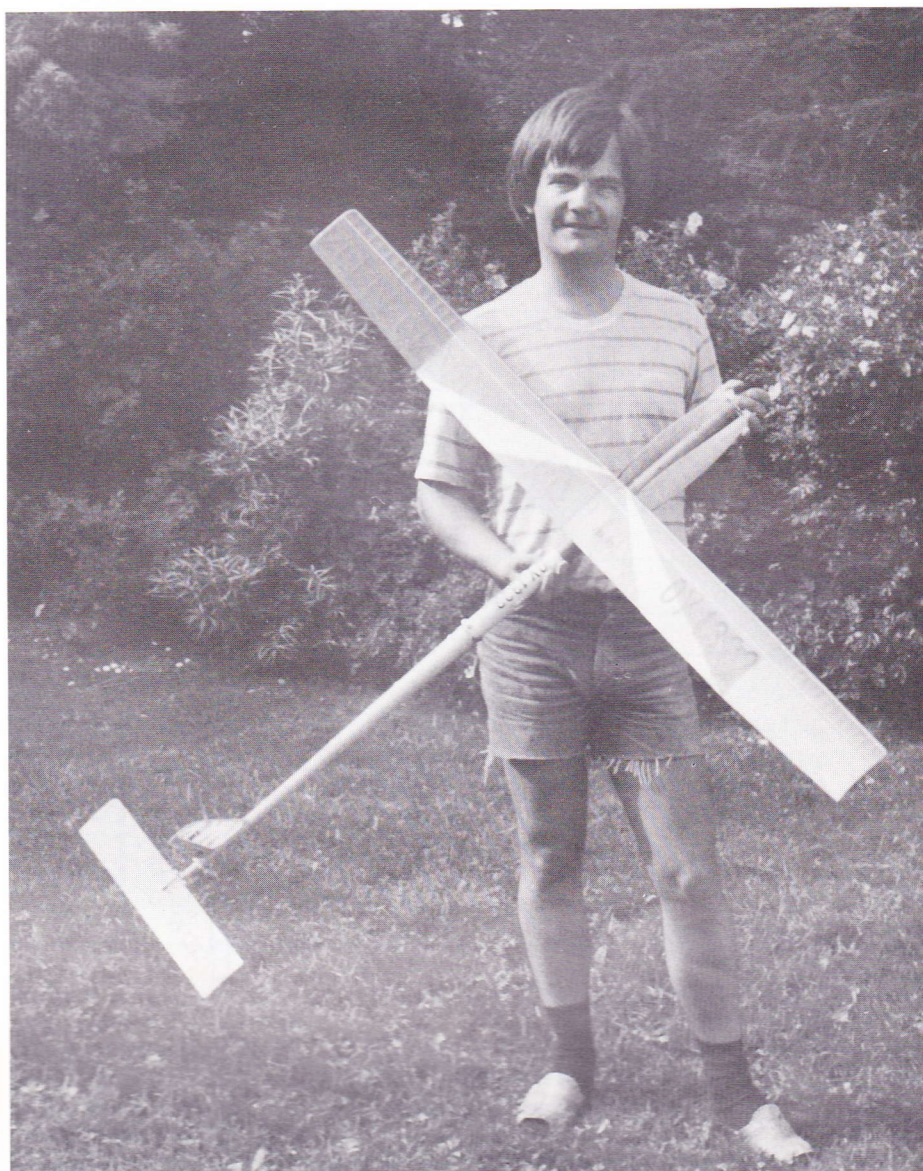
Jens med model nr. 20. På denne model er haleplanet papirkbæklædt
