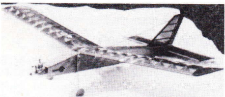
Lærken – en letbygget og stærk RC-begyndermodel med rolige og godmodige flyveegenskaber. Spændvidde 122 cm, længde 87 cm, motor 0,8 cm 3 med tank. RC-anlæg: 2 kanaler nødvendige. Byggesættet indeholder alle nødvendige trædele, styretøjsdele, hjul, fittings o.lign. Der mangler kun motor, lim og lak. Læs testen af Lærken i Modelflyve Nyt 3/83. Pris ..... kr. 295,-
