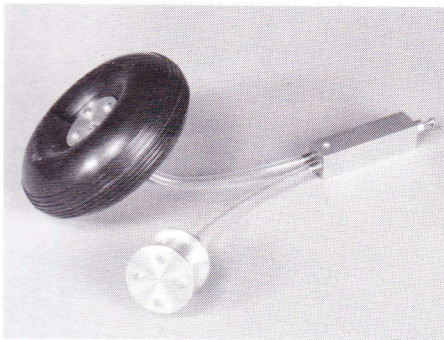
Tromlebremse
