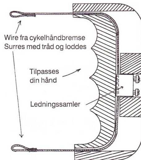
Fig. 5. Linestyre håndtag
