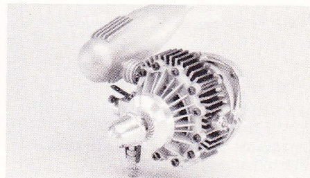
VANKEL MOTORER – Kammervolumen 4,97 cm 3 , direkte omløbs-indsugning, 2500 til 18000 o/min., 0,94 kW / 1,27 PS) ved 17000 o/min. .... kr. 1785,00
