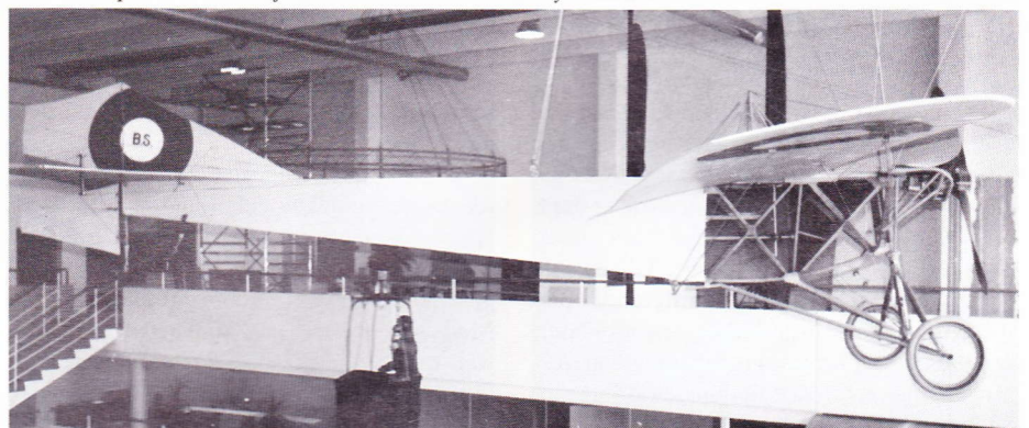
B&S monoplanet er nu et af klenodierne i Danmarks Flyvemuseum.
