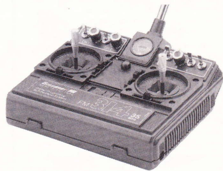
FM314 , 8-/14-kanals-FM-fjernstyringssæt for til- slutning af op til 7 rormaskiner. Efter eget valg plads til 2 moduler (omskiftere, proportional- eller Dual-Rate moduler). Servoreverse, længdestilbare styrehandtag med mekanisk trimning. Kort gummiantenne kan monteres. .... kr. 1225,-
