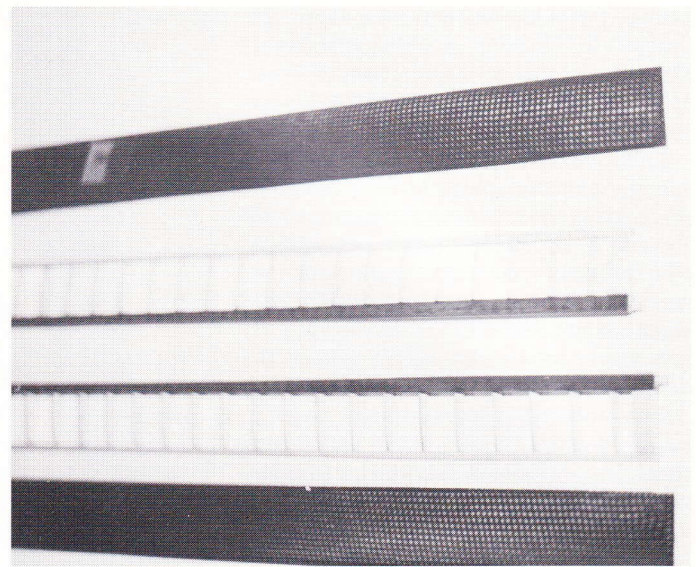
Fig. 4. (Til højre) De forreste dele af vingerne klar til pålimning af skaller. Det er ikke tydeligt på billedet, men fibrene i kulfiberen ligger 45/45 grader for endnu bedre vridningsstabilitet.
