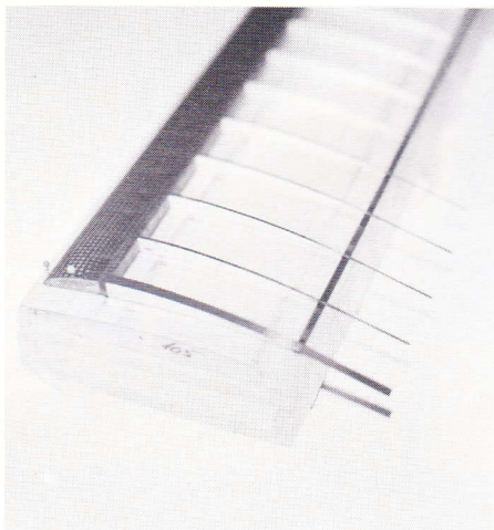
Fig. 8. Vingedelen er igen på jigger, denne gang til pålimning af capstrips på oversiden. Når dette arbejde er færdigt, er vingen »låst«, dvs. den kan ikke uden brutal vold vrides i en anden facon.
