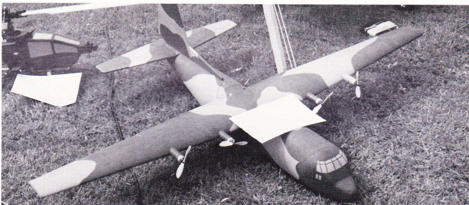
Hercules styrobomber, et herligt el-fly, der er forsynet med 4 stk. Speed 400 7,2V motorer, 8 stk. 1700 mha akkuer og 4 specielle Speed 400 propeller. Desuden benyttes ofte en fartregulator, da fuld kraft kun er nødvendigt i startfasen.
