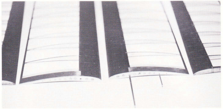
De færdige vingerødder. Det ses tydeligt, hvorledes capstripsene lapper ca. 3 mm ind over D-boxen.
