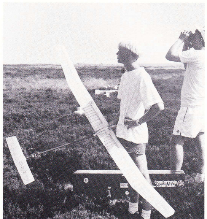
Ulrik Hansen med sin velflyvende F1A model. Profilerne i planet består af let balsa forstærket med 0,2 mm kulfiber på over- og underside. Det ses som mørke tværstriber på planet.
