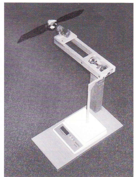
Billede 3: Teststand til måling af udgangseffekt.
