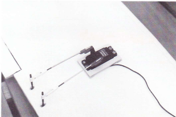
Krængerorsservoene. V-formen på servohornene giver en vis differentiering, dvs. større udslag opad end nedad.
