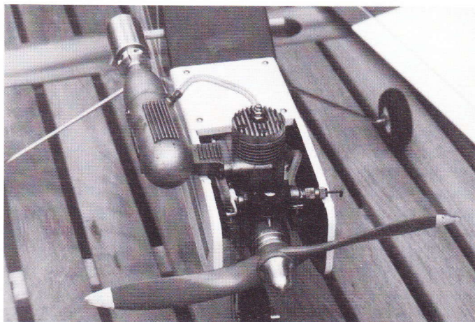
En Irvine .46 på det fiks motorfundament. "Mouse" efterdæmperen bringer støjen ned på et acceptabelt niveau.
