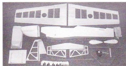
CAP 232 i hhv. elektroversionen (øverst) og brændstofversionen. Bemærk, at kroppen er med aftageligt cowl.
