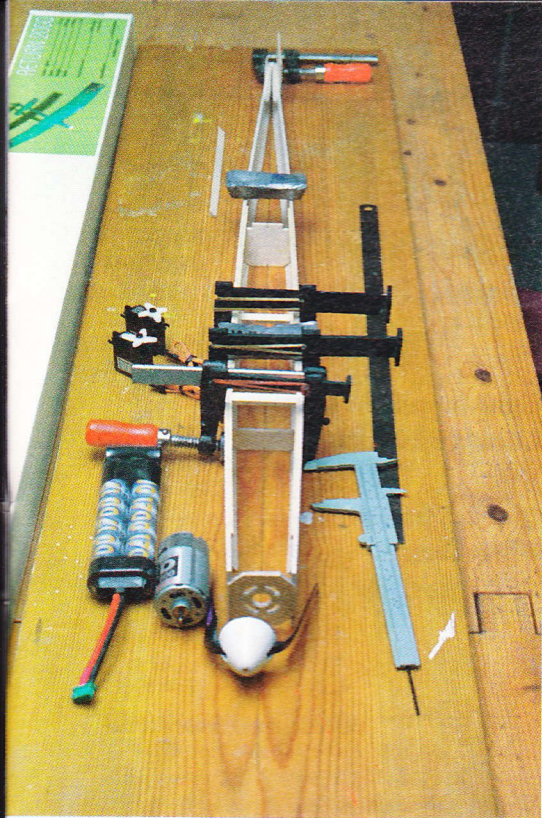
Kroppen samles på byggebrættet. Motorspantet er reduceret i højde og bredde, og der er udskåret kølehuller til motoren. Jeg har kontrolleret, at der er plads til motoren, og at det er muligt at udskifte batteriet.
