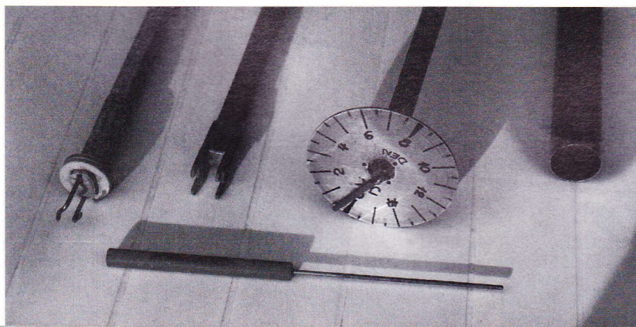
9. Ladestok, momentmåler og beskyttelsesrør i nærbillede. Dimsen længst til venstre er en "gummimotorudgraver" (når motoren sprænges, og det meste af den bliver inde i selv modellens krop.) Pinden med plasthåndtaget foran de øvrige ting er til hjælp ved montering af propellen efter optrækket.
