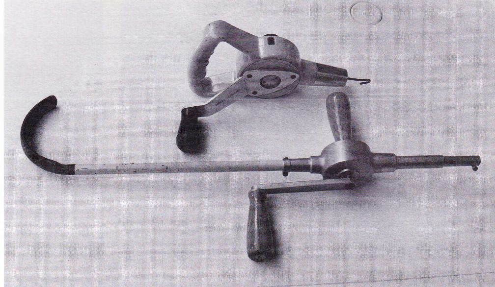
7. To forskellige optrækkere. Den korte har tjent forfatteren i mere end 25 år! Det er en ombygget boremaskine, hvor krogerne af hensyn til risikoen for metaltræthedbrud udskiftes med jævne mellemrum. Den anden er specielt lavet til optræk af gummimotorer og kommer fra Ukraine. Den er meget solidt lavet og forsynet med paraplyhåndtag, der sættes om overarmen, når man trækker op. Pris ca. 900 kroner.
