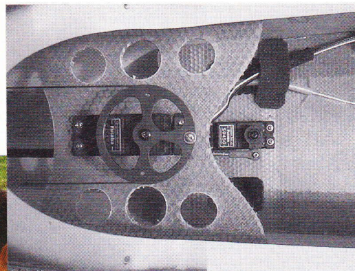
De lette Nomex plader, her med glasvæv. De bruges meget til servoplader. Begge servoer er de nye digitale. Rorhornet er også her lilla eloxeret aluminium.
