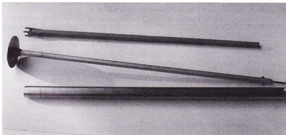
8. Ladestok, momentmåler og beskyttelsesrør - se i øvrigt også fig.
