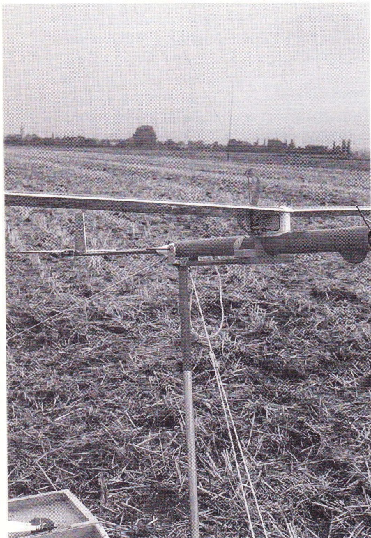
12. Tre solide barduner (den ene kan desværre ikke rigtig ses på dette billede) og meget kraftige teltpløkke holder optræksstativet på plads. Der er store kræfter i sving, når man trækker op.
