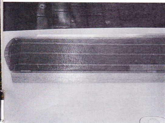
Krængerorene holdes på plads af små træstykker, inden de limes på med tape.
