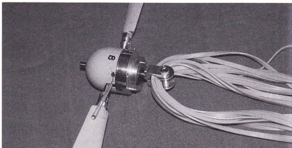
6. Her ses gummimotoren sat igennem bobbinen (trissen) på propelaggregatet.
