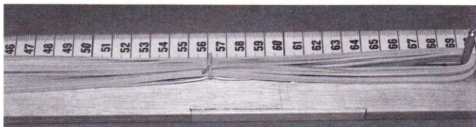
4. Et bræt til oplægning af gummimotorer. Pinden til højre løber i et stykke gardinstang, så den kan justeres med henblik på at få alle strenge lige lange. En lille nylonkrue låser i den ønskede position. Linealen er et stykke målebånd, der er limet fast på brættet, så man kan kontrollere længden af motorerne.
