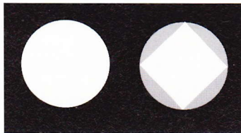
Fig. 2 Til venstre ses okularet (tættest ved øjet) fra en god kikkert. Skyggerne på det andet er tegn på en dårlig optik.
