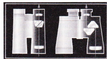
Fig. 1 Kikkerten til venstre har tagprismer og den til højre porroprismer.
