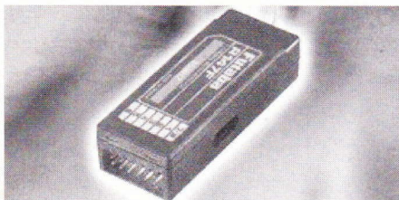
R-147 F MODTAGER ..... Kr. 795,- 7 kanaler, FM 35 eller FM 40 - mål 24,2x17,6x64 mm - Vægt 26 g
