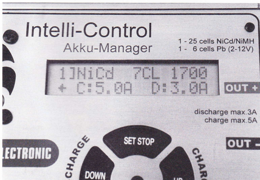
Dette display viser et ladeprogram til en 7 celled Ni cd akku på 1.700 mAh. Den skal lades med 5 A og aflades med 3 A.
