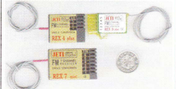
Jeti 4k plus, 4 kanaler, 9 gram 275,- Jeti 5k plus, 5 kanaler, 8 gram 295,- Jeti 7k mini, 7 kanaler, 15 gram 350,- Jeti 18 A fartregulator fra 250,- Jeti 35 A fartregulator fra 325,- Jeti mini-charger 4-7(8) celler kun 225,- Jeti DIS10/15 afader 6-15 celler kun 225,-
